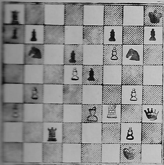
7. Maroczy - Forster
